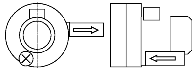
Fig. 3: Turbinas de canal lateral de doble etapa (dos rodetes en serie) Double stage side channel blower (2 impellers in serial) Series: ASCxxxx-2S... Двухступенчатые турбокомпрессоры (два рабочих колеса расположением напорного патрубка перпендикулярно центральной оси турбокомпрессора) Серии: ASCxxxx-2S....
