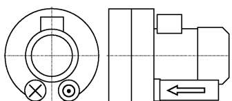
Fig. 2: Turbinas de canal lateral de doble etapa (2 rodetes en paralelo) Double stage side channel blower (2 impellers in parallel) Series: ASCxxxx-2P... Двухступенчатые турбокомпрессоры (2 рабочих колеса, патрубки расположены параллельно) Серии: ASCxxxx-2P....
