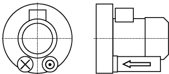
Fig. 1: Turbinas de canal lateral de simple etapa (1 rodete) Single stage side channel blower (1 impeller) Series: ASCxxxx-1M... Одноступенчатые турбокомпрессоры (1 рабочее колесо) Серии: ASCxxxx-1M....
